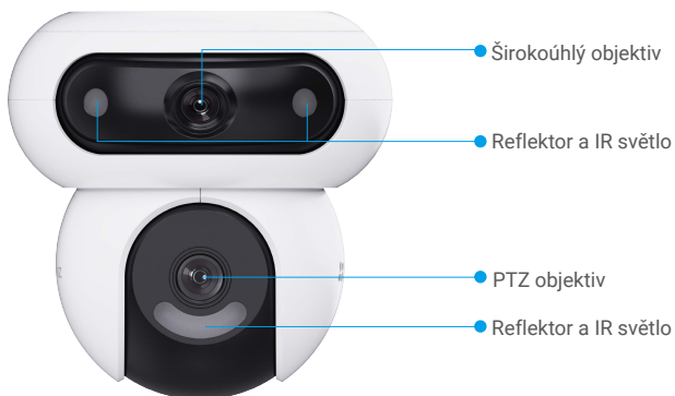
Čelní pohled
